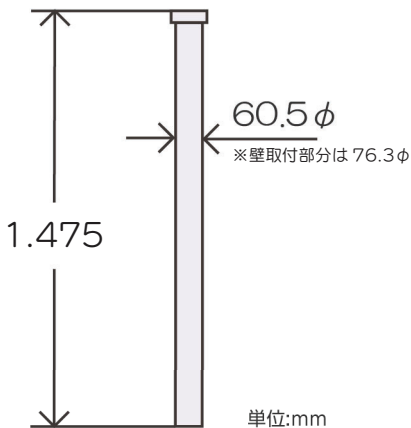
横断面図
