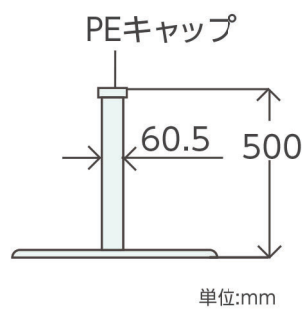
横断面図
