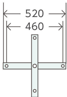
上面図
