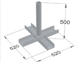
施工イメージ
