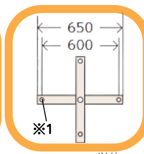
上面図
